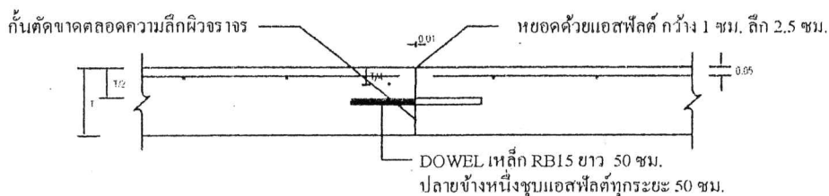
รอยต่อระหว่างก่อสร้าง (กรณีมีการหยุด)
