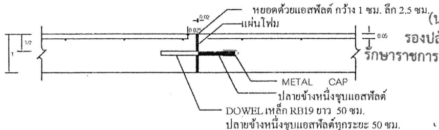
รอยต่อเพื่อการขยายตัวทุกระยะ 30 เมตร
