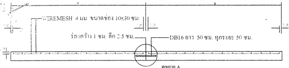
การเสริมเหล็กถนนคอนกรีตเสริมเหล็ก
