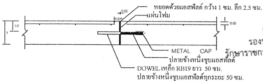
รอยต่อเพื่อการขยายตัวทุกระยะ 30 เมตร
