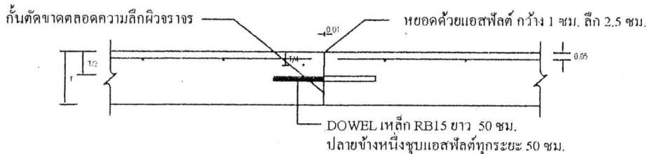
รอยต่อระหว่างก่อสร้าง (กรณีมีการหยุดเท)
