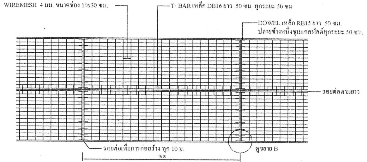
แปลนแสดงการเสริมเหล็กถนนคอนกรีตเสริมเหล็ก
