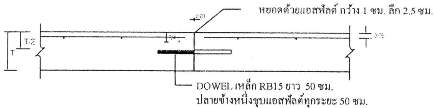
รอยต่อระหว่างแผ่นระยะ 10 เมตร
