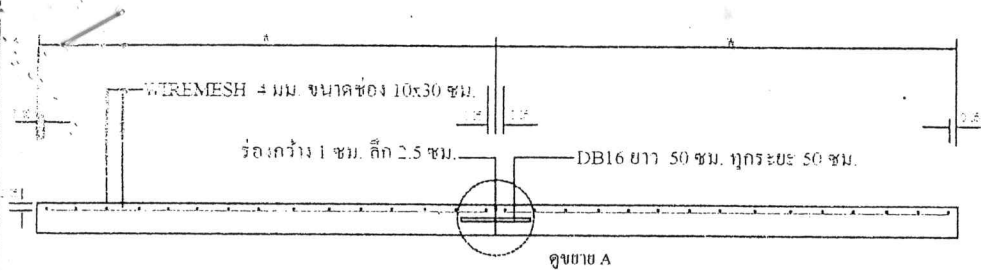
การเสริมเหล็กถนนคอนกรีตเสริมเหล็ก
