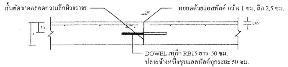
รอยต่อระหว่างก่อสร้าง (กรณีมีการหยุด) หมายเหตุ แบบนี้เป็นแบบตัดออกจากแบบมาตรฐานถนน คลส. ของกรมทางหลวงชนบท
