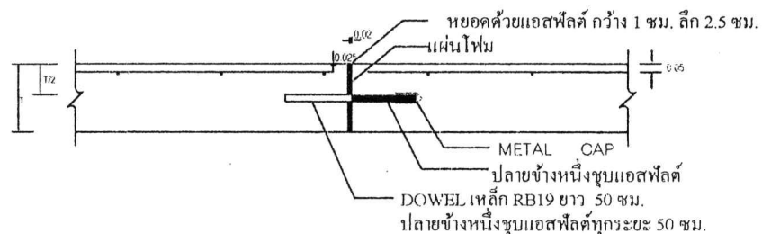
รอยต่อเพื่อการขยายตัวทุกระยะ 30 เมตร NOT TO SCALE
