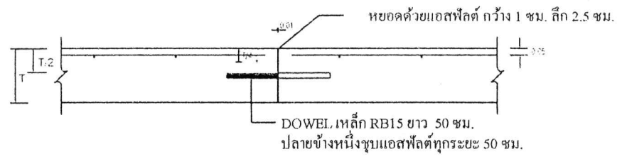
รอยต่อระหว่างแผ่นระยะ 10 เมตร NOT TO SCALE
