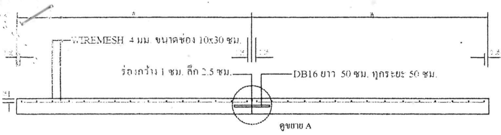
การเสริมเหล็กถนนคอนกรีตเสริมเหล็ก NOT TO SCALE
