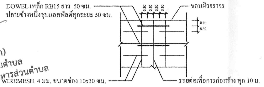
แปลนแสดงการเสริมเหล็กถนนคอนกรีตเสริมเหล็ก NOT TO SCALE
